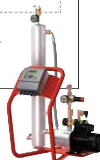
Вакуумный деаэратор reflex 'servitec' в стандартном исполнении
