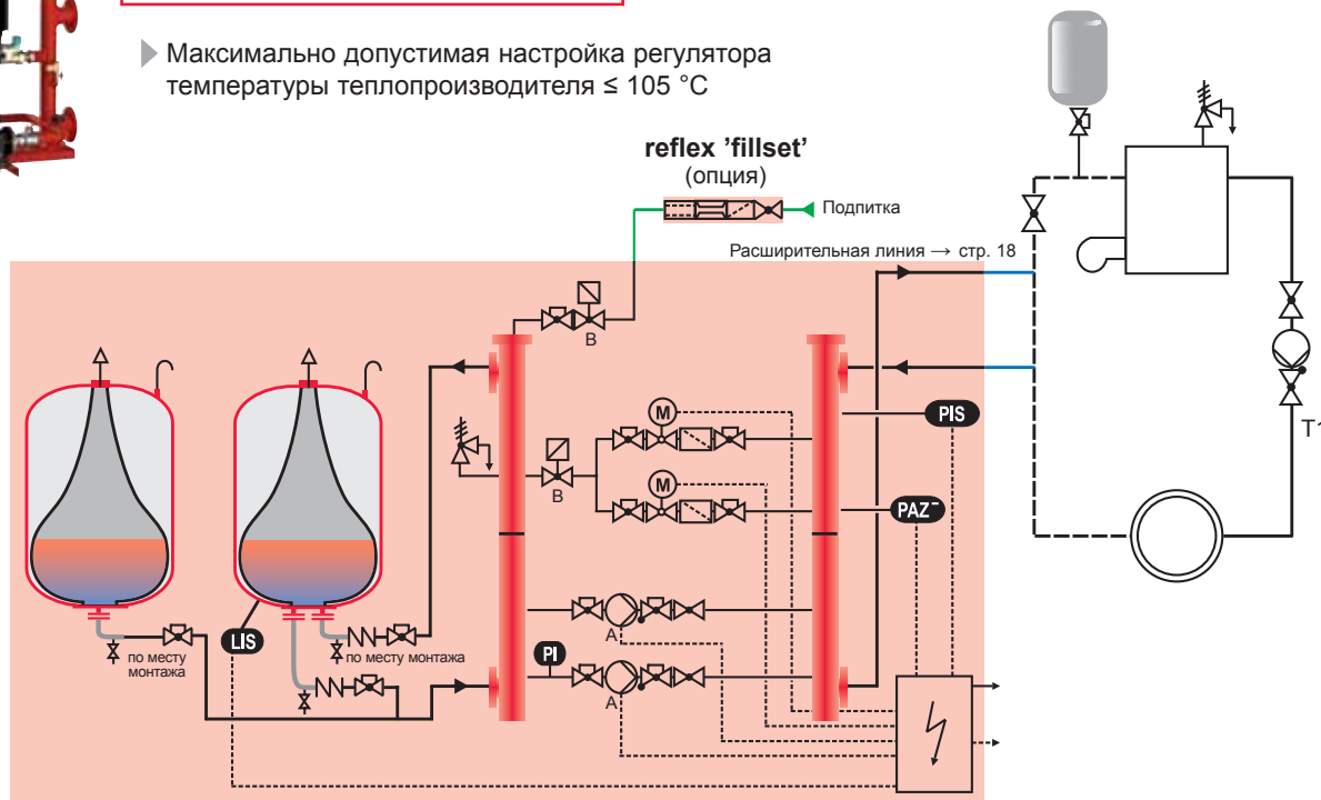
Дополнительная ёмкость GF (опция)
